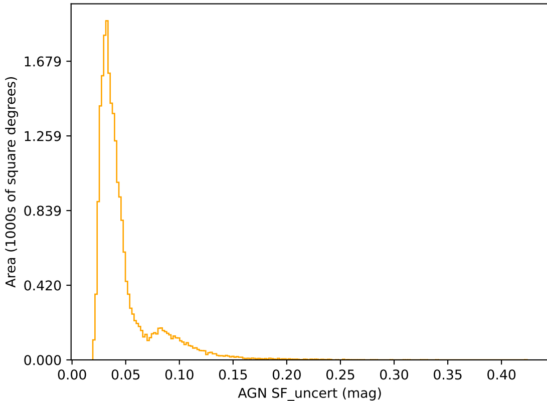
weather_cloudso36v3.4_10yrs r band: AGN SF_uncert
