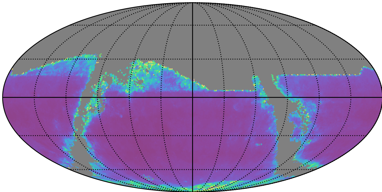
weather_cloudso36v3.4_10yrs i band: AGN SF_uncert
