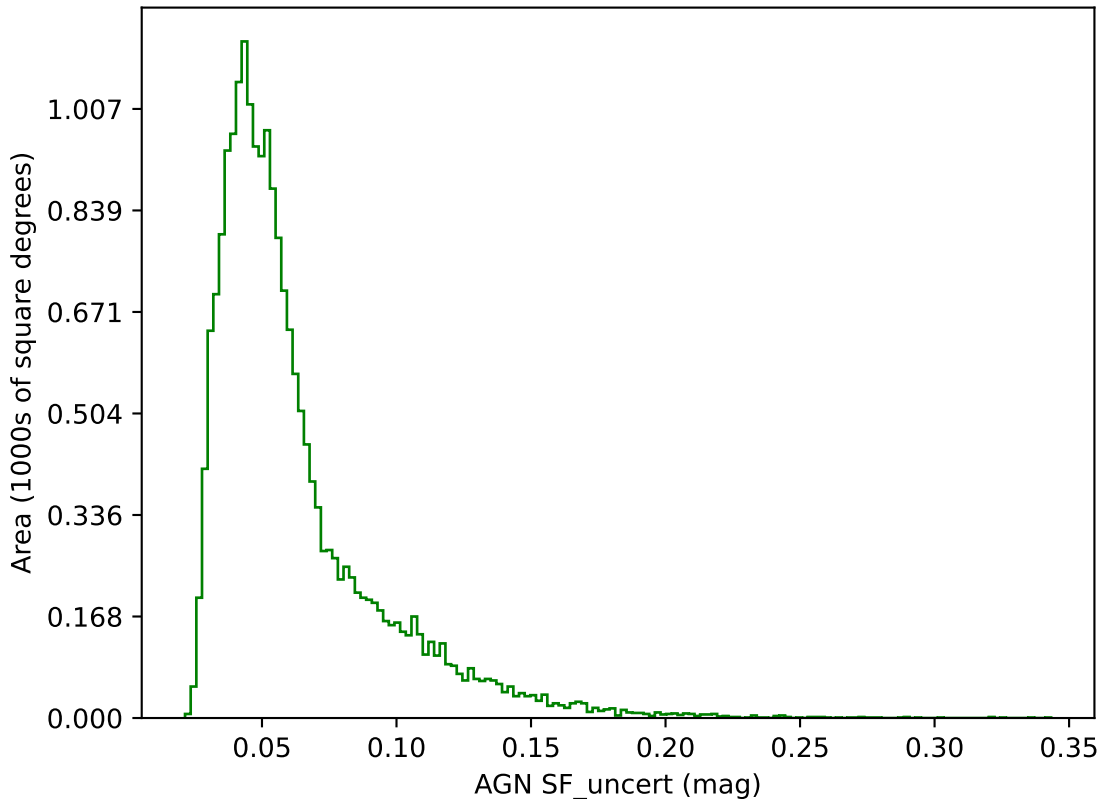
weather_cloudso36v3.4_10yrs g band: AGN SF_uncert
