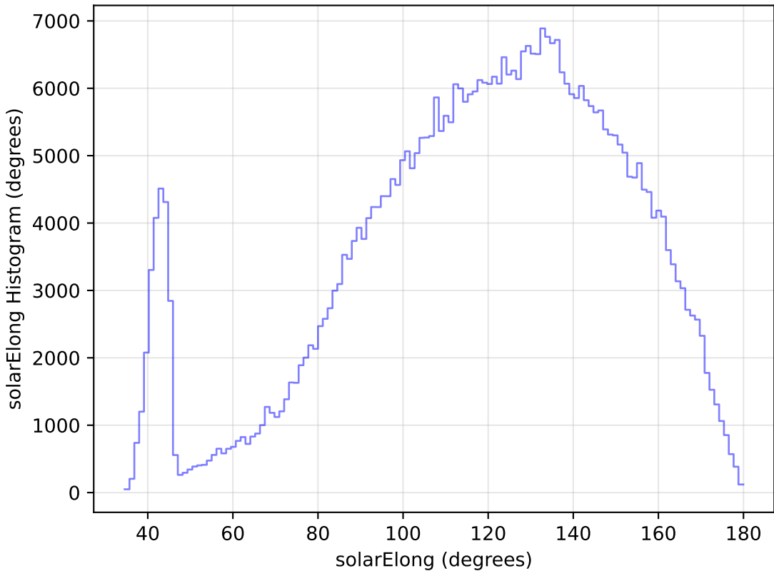
weather_cloudso36v3.4_10yrs WFD z band: solarElong Histogram
