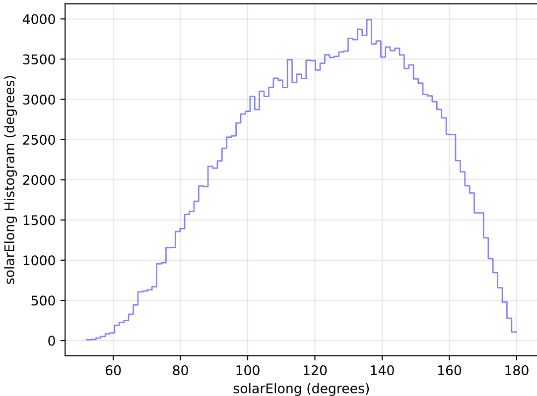
weather_cloudso36v3.4_10yrs WFD g band: solarElong Histogram
