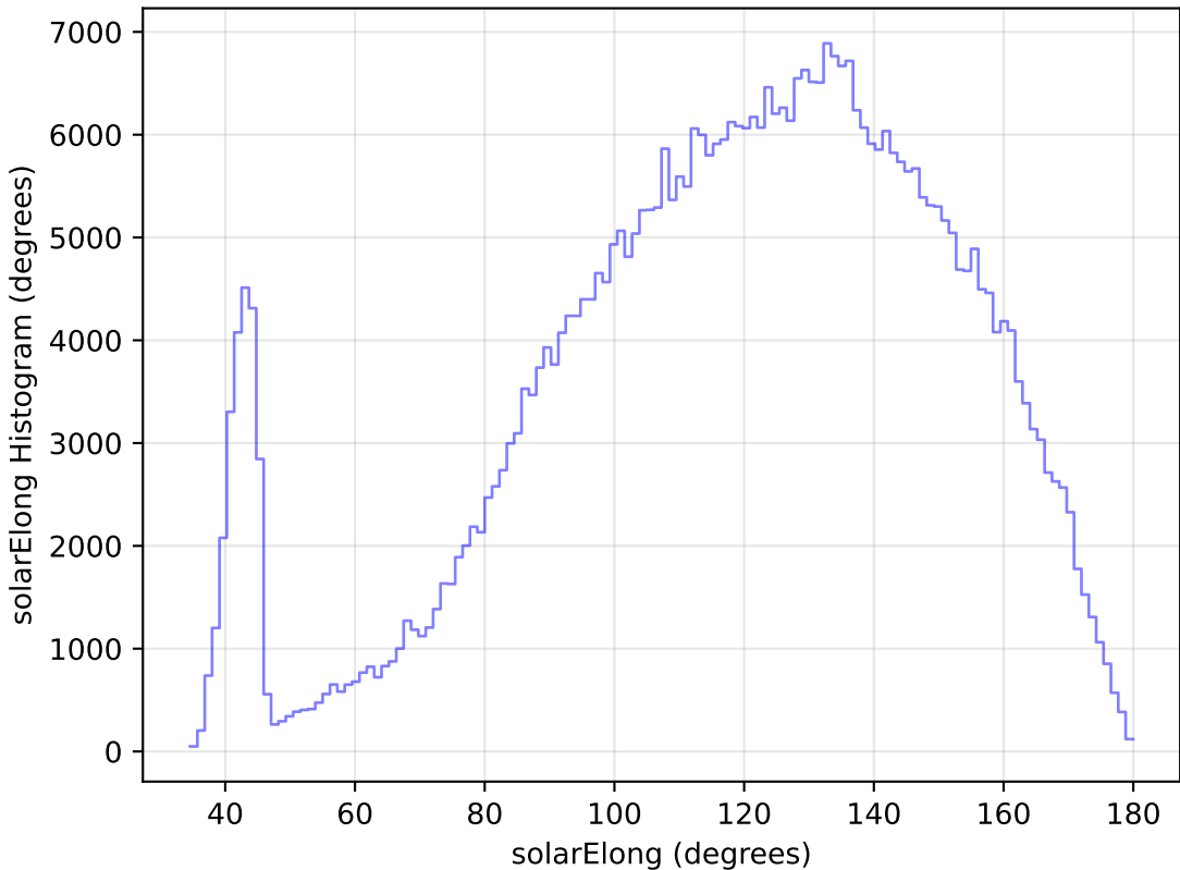
weather_cloudso36v3.4_10yrs All sky z band: solarElong Histogram
