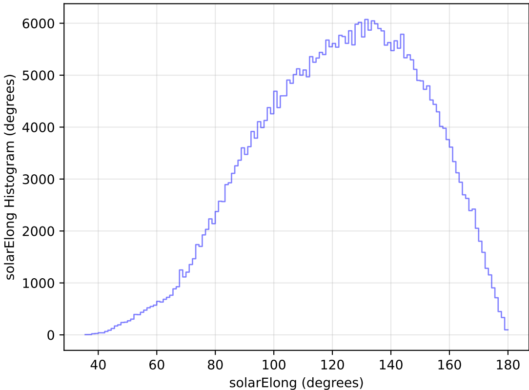
weather_cloudso36v3.4_10yrs All sky y band: solarElong Histogram
