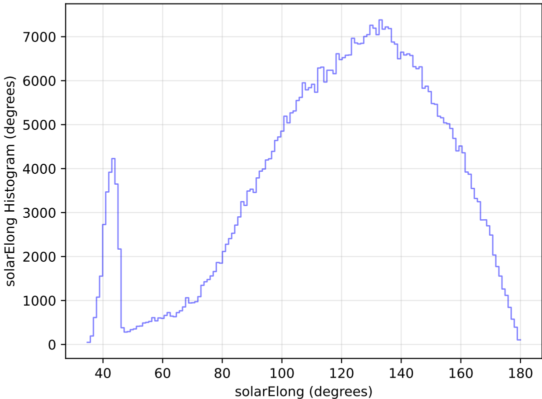
weather_cloudso36v3.4_10yrs All sky i band: solarElong Histogram
