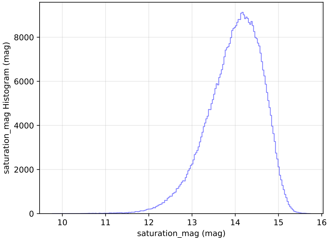
weather_cloudso36v3.4_10yrs WFD z band: saturation_mag Histogram
