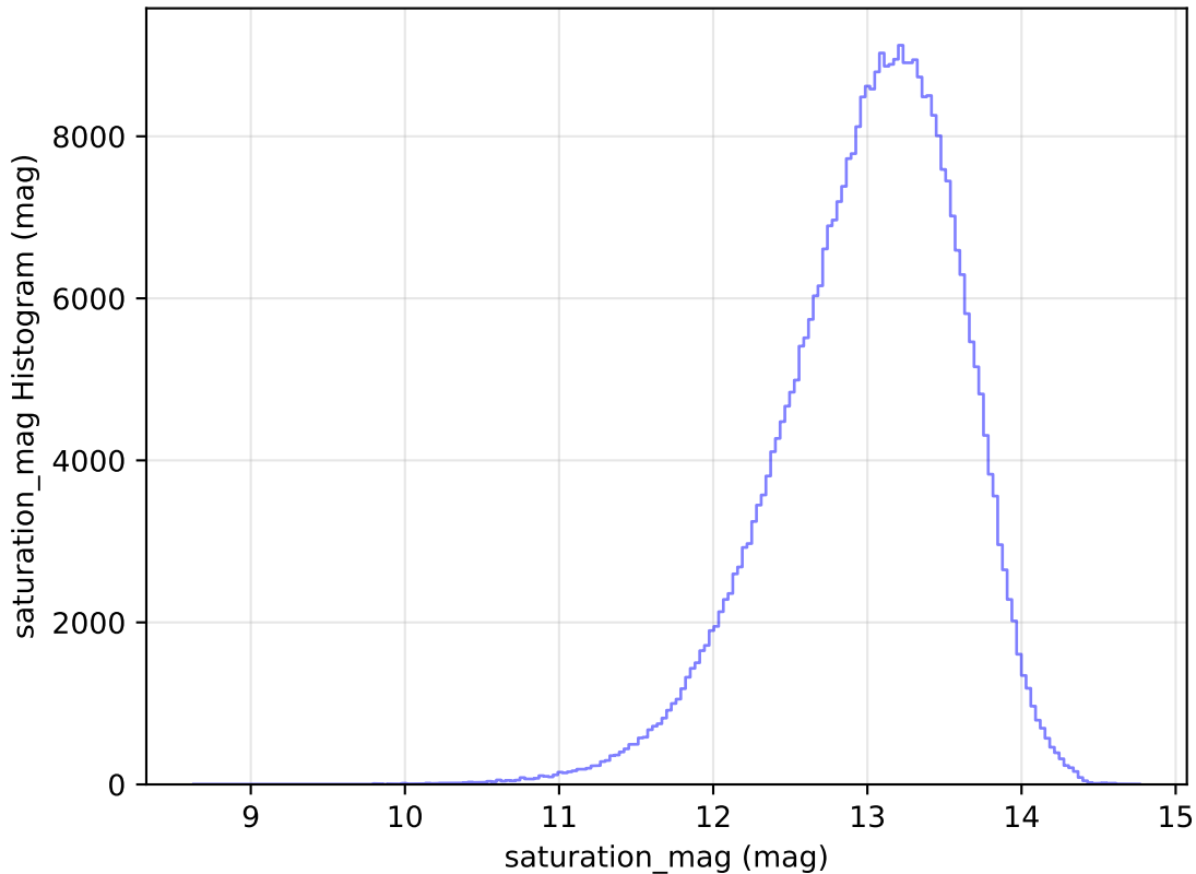
weather_cloudso36v3.4_10yrs WFD y band: saturation_mag Histogram
