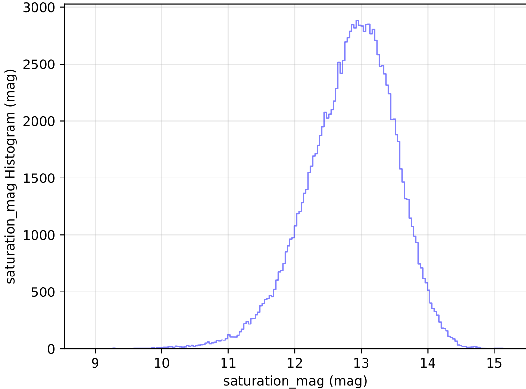
weather_cloudso36v3.4_10yrs WFD u band: saturation_mag Histogram
