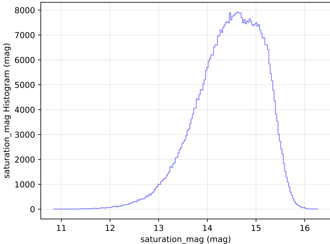
weather_cloudso36v3.4_10yrs WFD r band: saturation_mag Histogram
