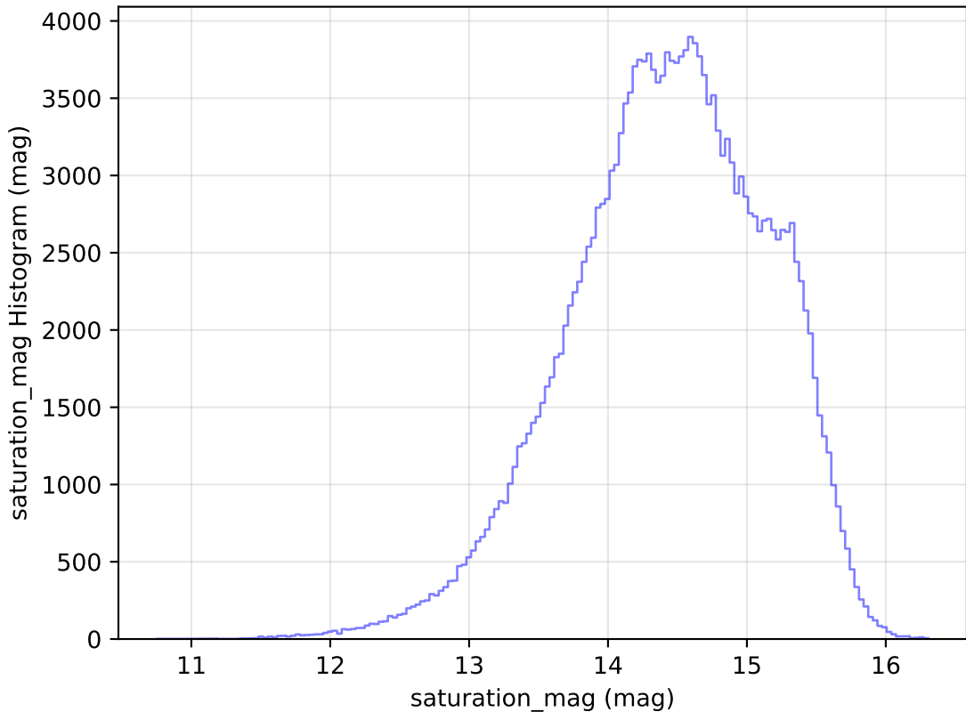
weather_cloudso36v3.4_10yrs WFD g band: saturation_mag Histogram
