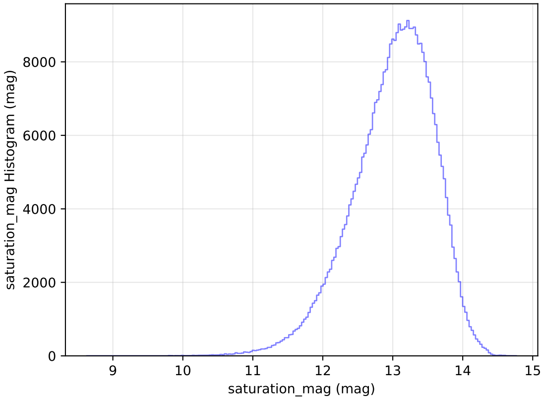
weather_cloudso36v3.4_10yrs All sky y band: saturation_mag Histogram
