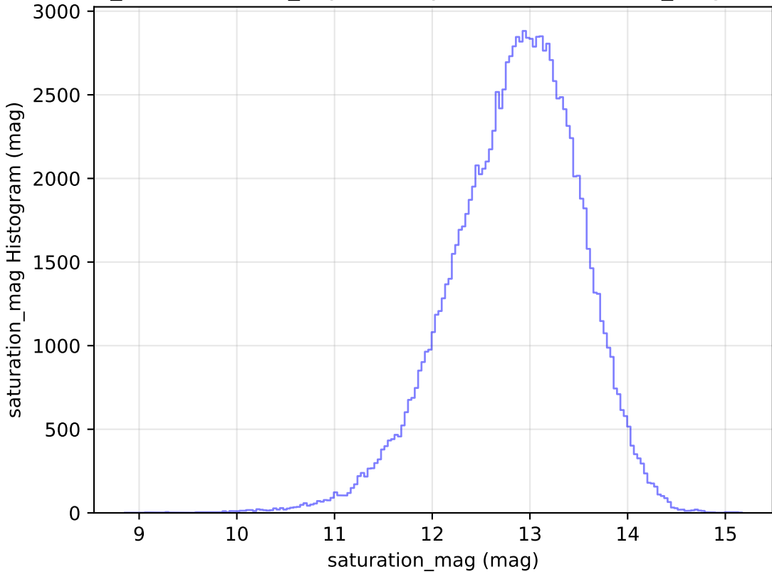
weather_cloudso36v3.4_10yrs All sky u band: saturation_mag Histogram
