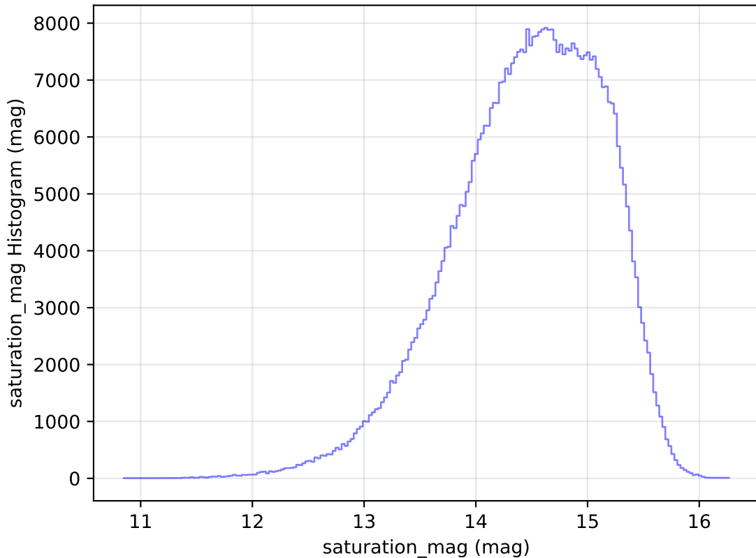
weather_cloudso36v3.4_10yrs All sky r band: saturation_mag Histogram
