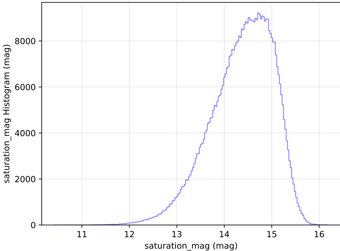
weather_cloudso36v3.4_10yrs All sky i band: saturation_mag Histogram
