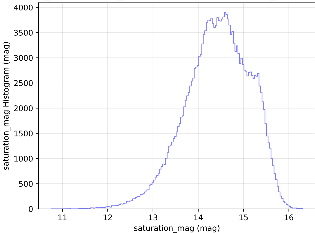
weather_cloudso36v3.4_10yrs All sky g band: saturation_mag Histogram
