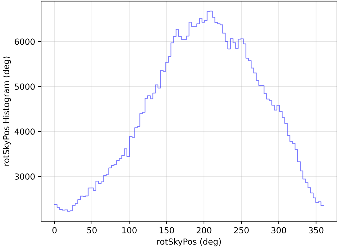
weather_cloudso36v3.4_10yrs WFD z band: rotSkyPos Histogram
