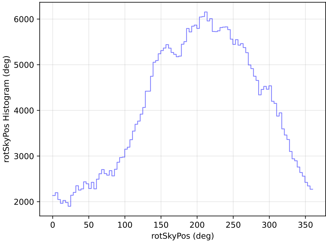
weather_cloudso36v3.4_10yrs WFD y band: rotSkyPos Histogram
