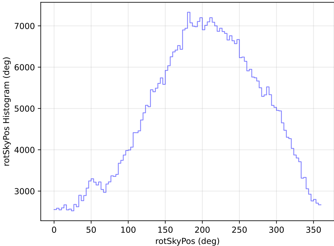
weather_cloudso36v3.4_10yrs WFD i band: rotSkyPos Histogram
