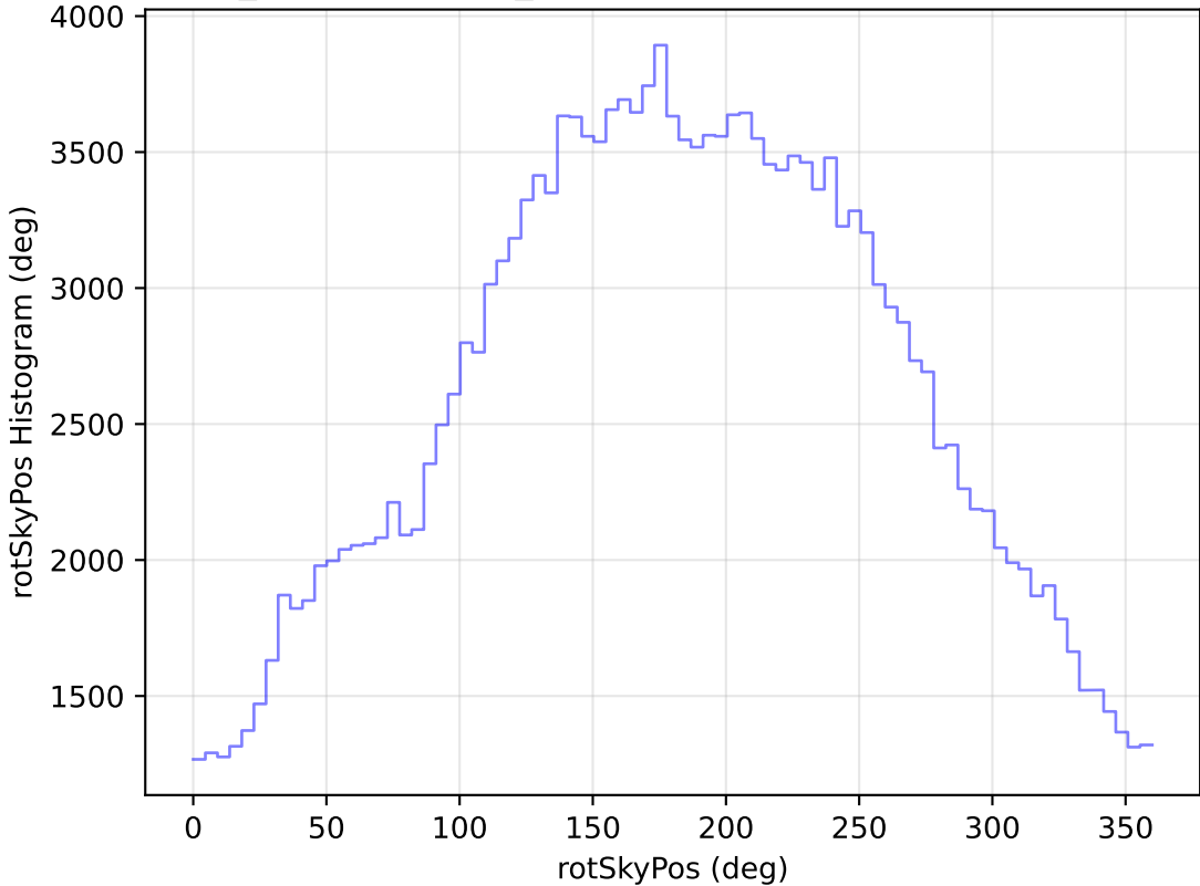
weather_cloudso36v3.4_10yrs WFD g band: rotSkyPos Histogram
