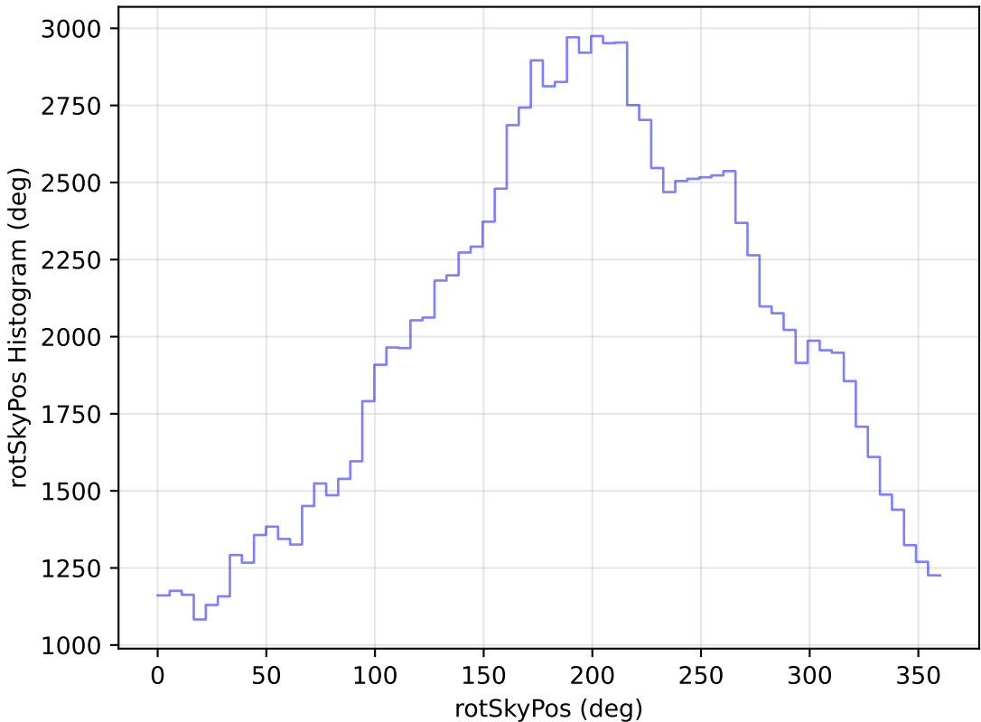
weather_cloudso36v3.4_10yrs All sky u band: rotSkyPos Histogram
