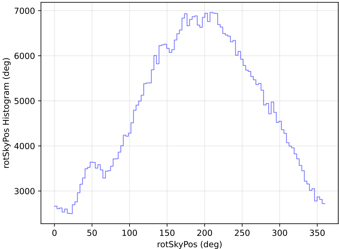
weather_cloudso36v3.4_10yrs All sky r band: rotSkyPos Histogram
