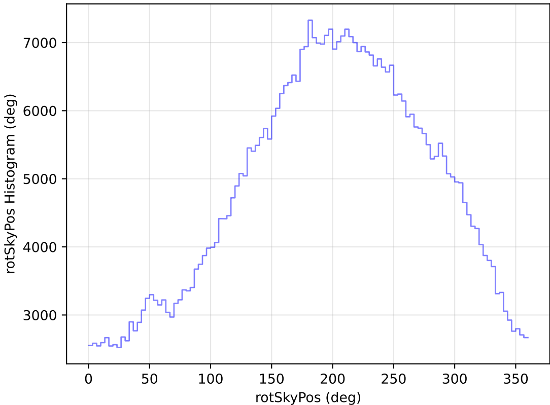
weather_cloudso36v3.4_10yrs All sky i band: rotSkyPos Histogram
