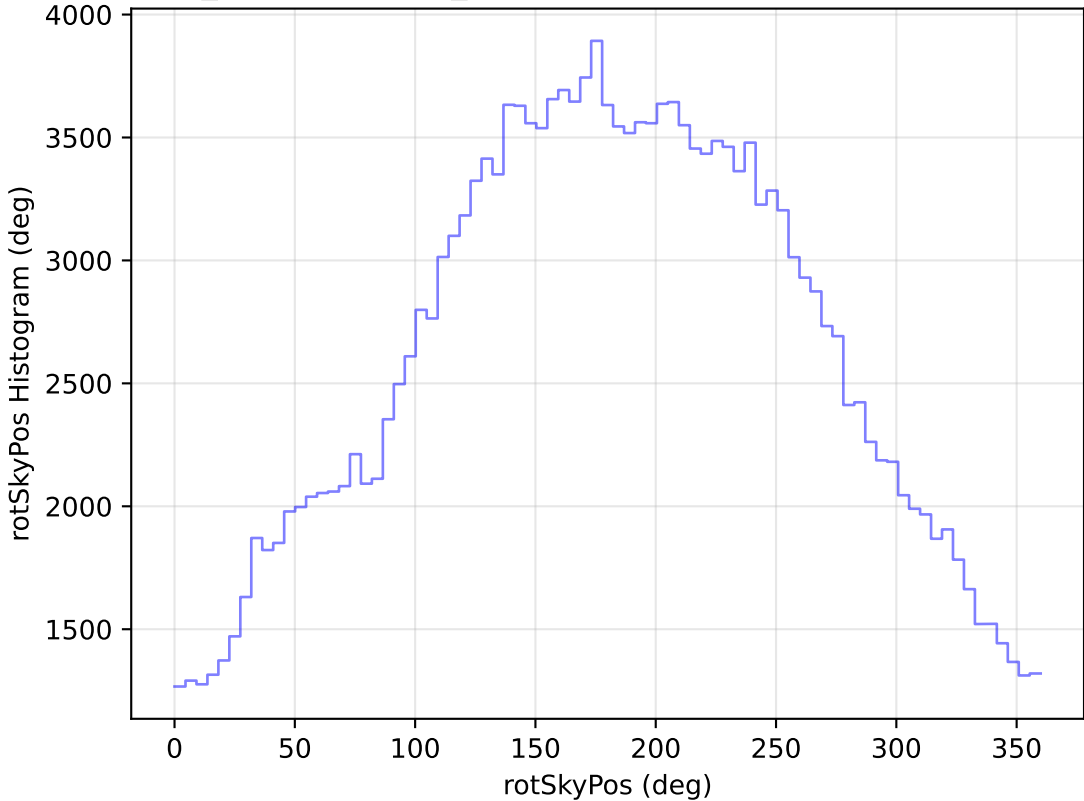
weather_cloudso36v3.4_10yrs All sky g band: rotSkyPos Histogram
