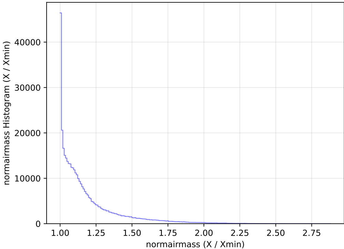
weather_cloudso36v3.4_10yrs WFD y band: normairmass Histogram
