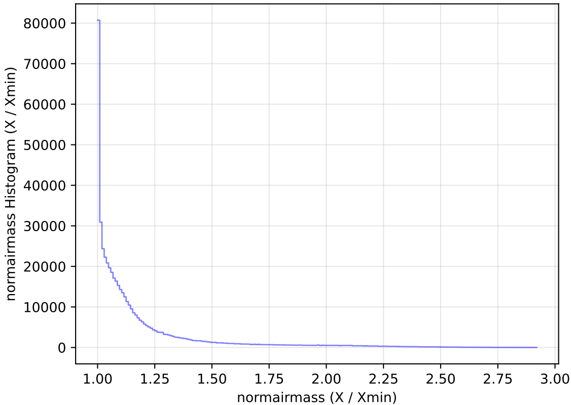
weather_cloudso36v3.4_10yrs WFD i band: normairmass Histogram
