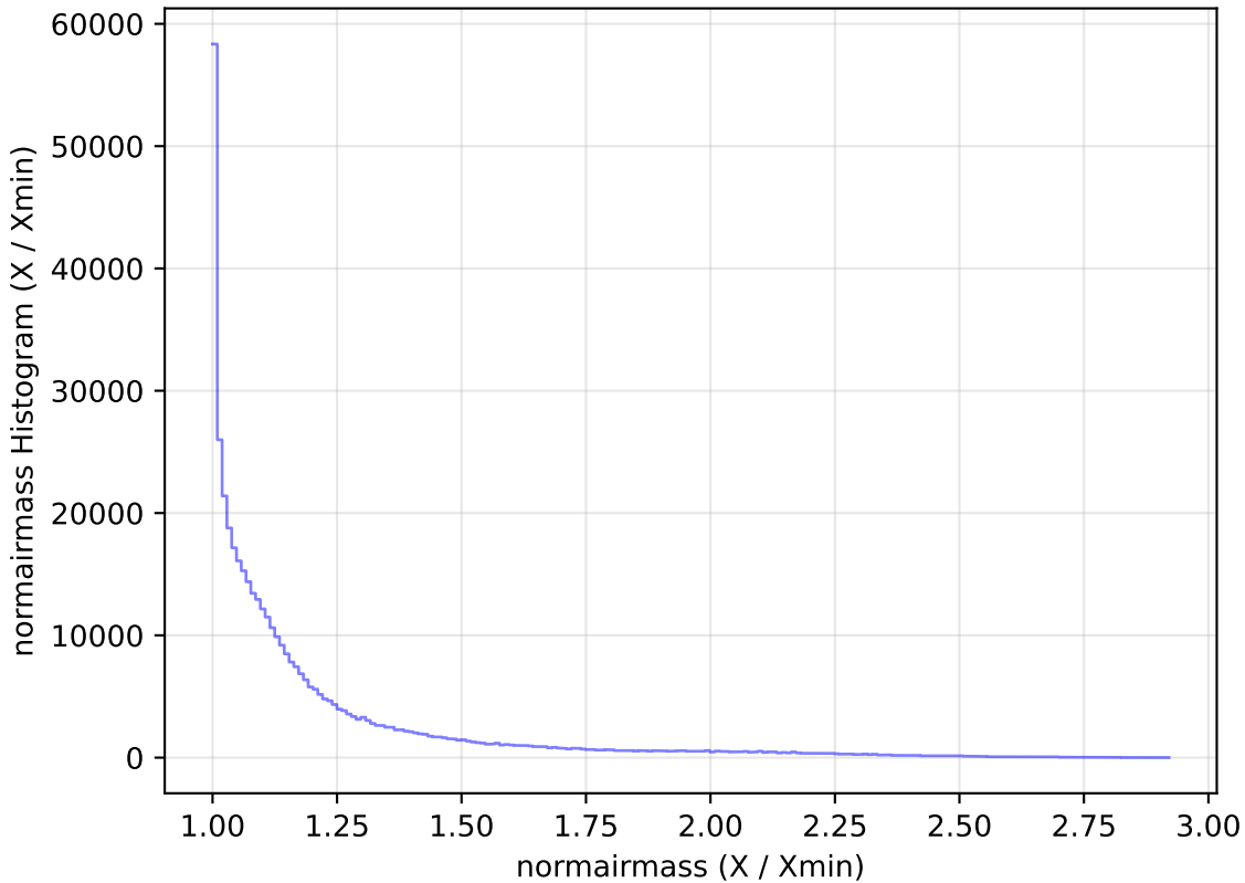
weather_cloudso36v3.4_10yrs All sky z band: normairmass Histogram
