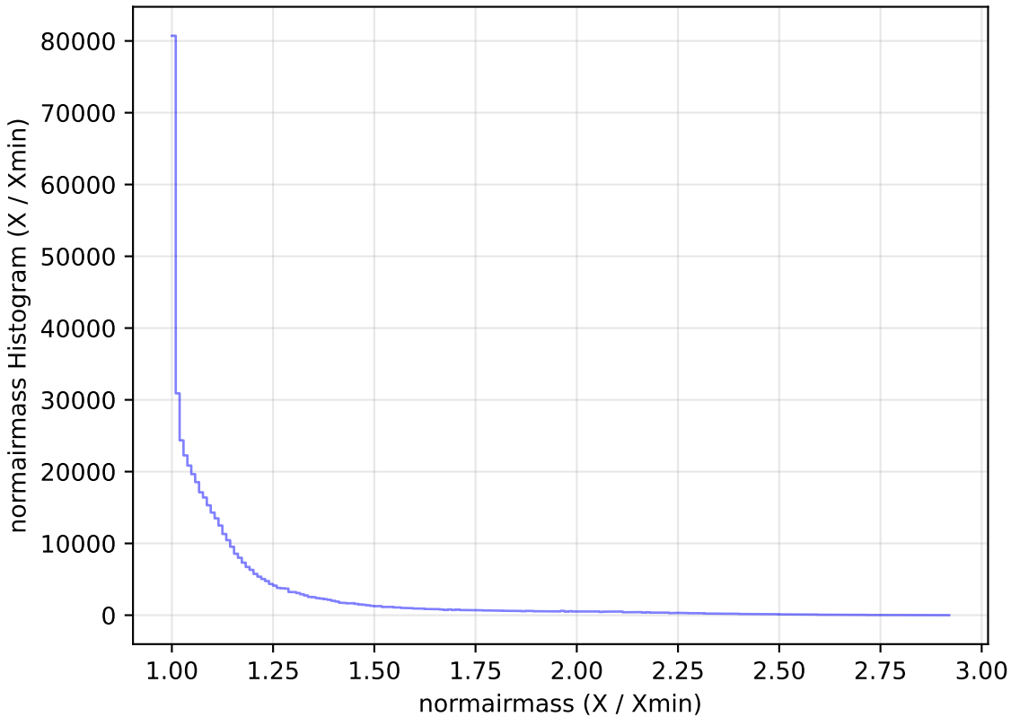
weather_cloudso36v3.4_10yrs All sky i band: normairmass Histogram
