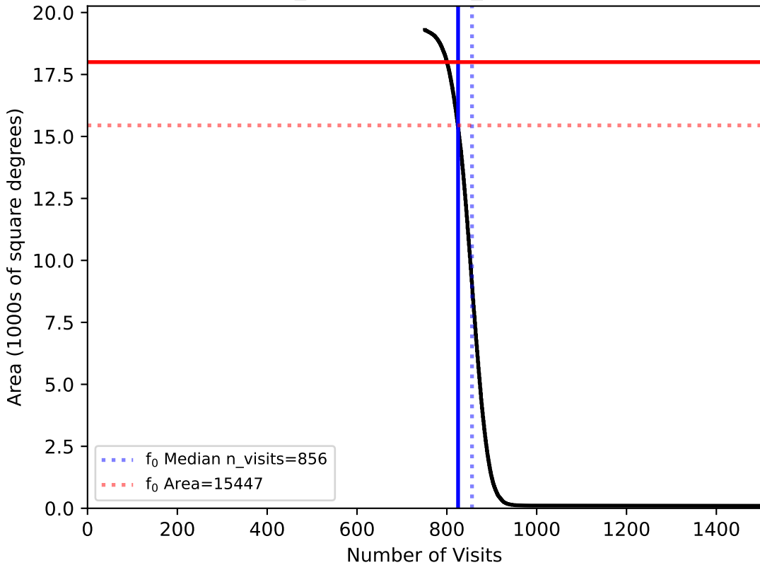
weather_cloudso36v3.4_10yrs WFD: f0
