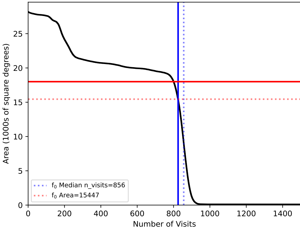
weather_cloudso36v3.4_10yrs All sky: f0
