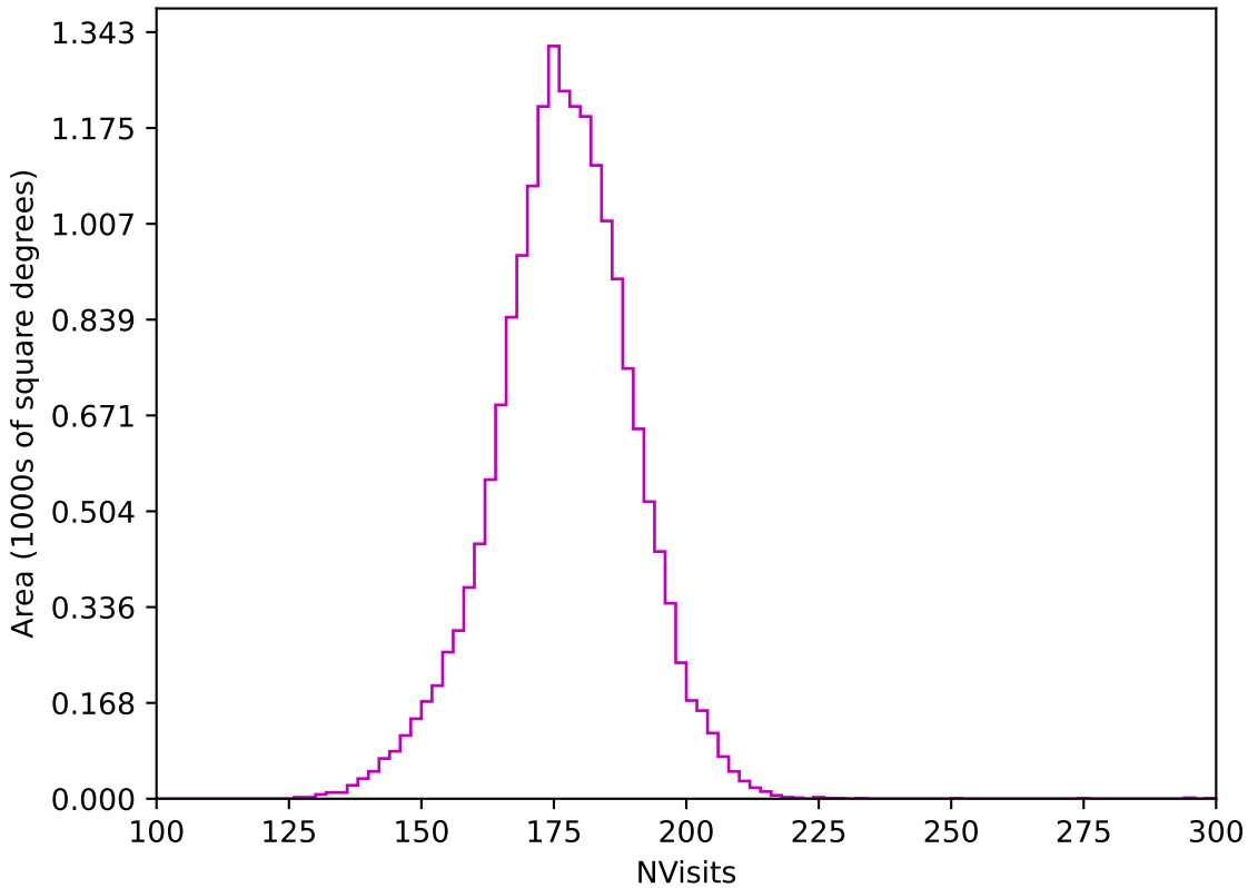
weather_cloudso36v3.4_10yrs WFD z band: NVisits
