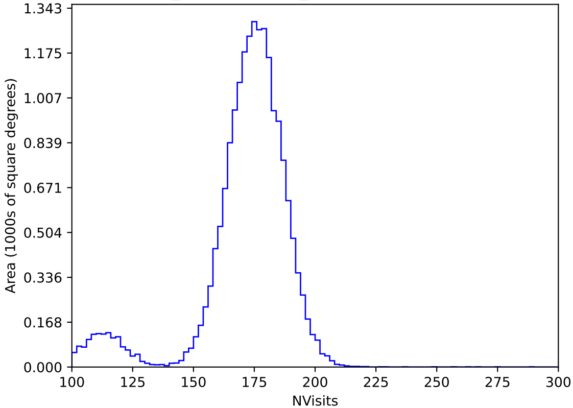
weather_cloudso36v3.4_10yrs WFD y band: NVisits
