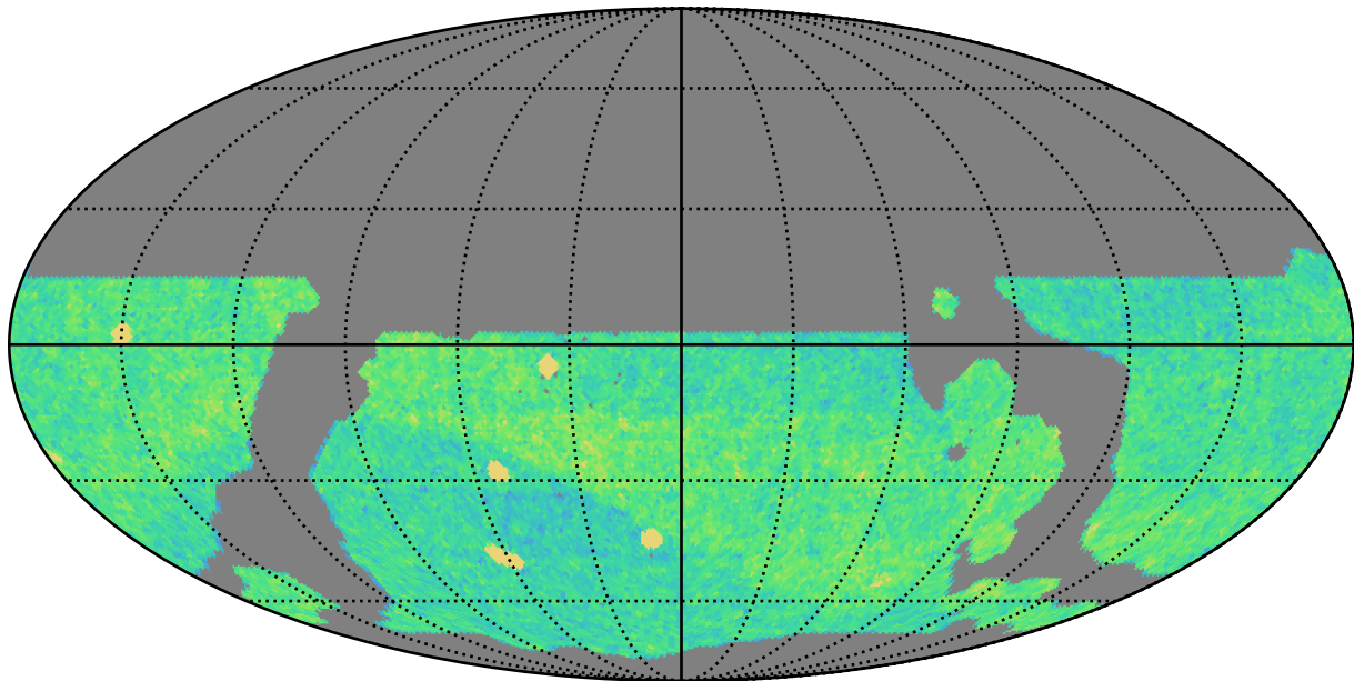
weather_cloudso36v3.4_10yrs WFD i band: NVisits
