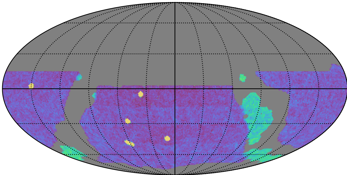
weather_cloudso36v3.4_10yrs WFD g band: NVisits
