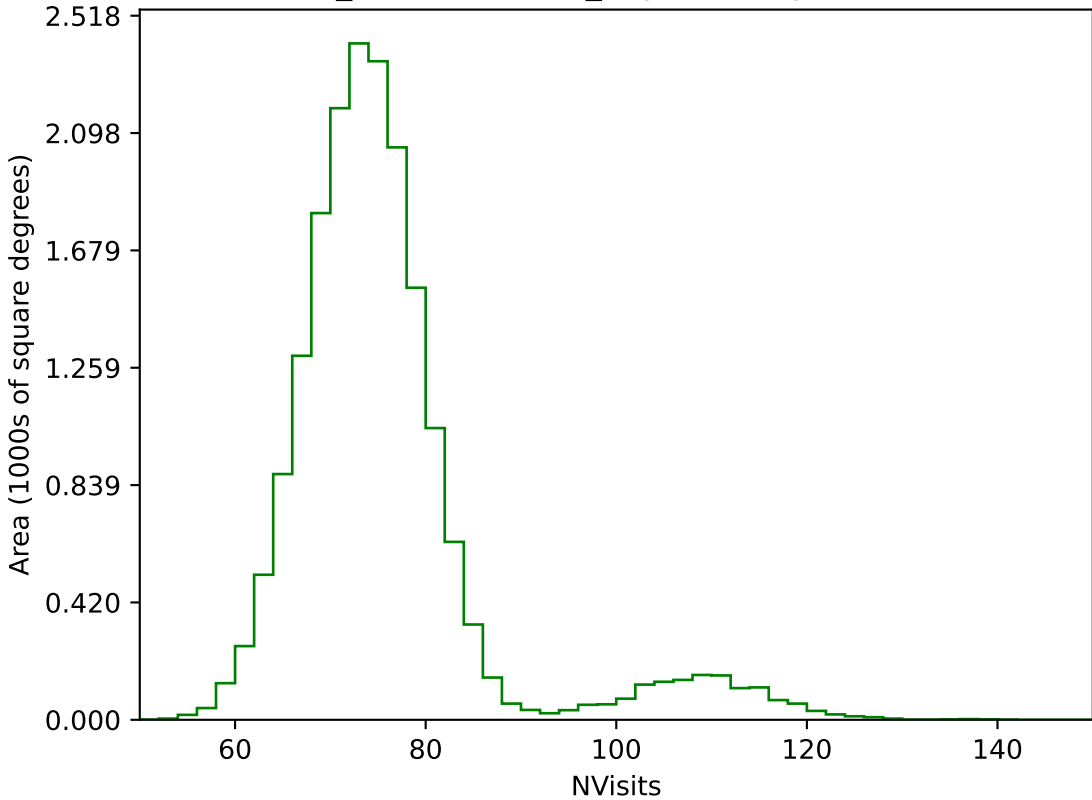
weather_cloudso36v3.4_10yrs WFD g band: NVisits
