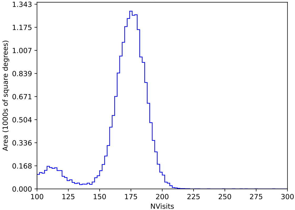
weather_cloudso36v3.4_10yrs All sky y band: NVisits
