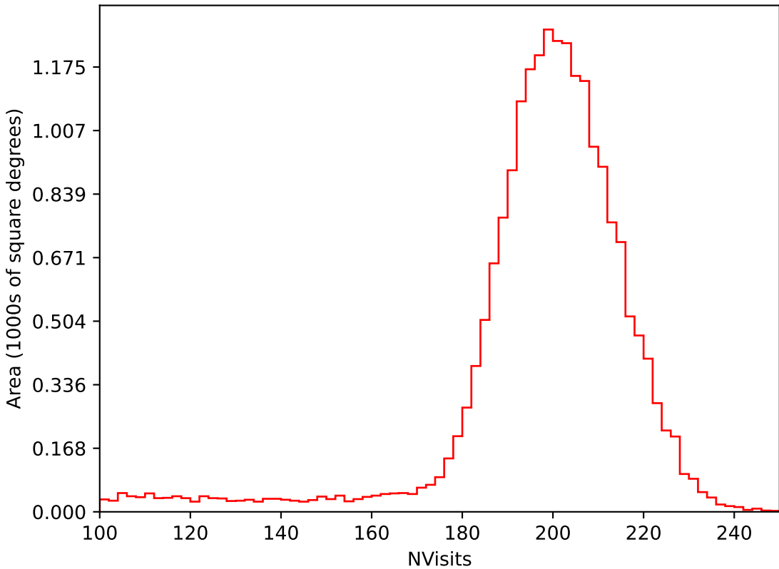
weather_cloudso36v3.4_10yrs All sky i band: NVisits
