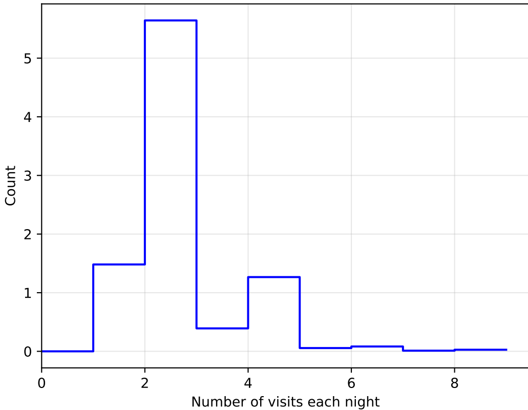
1e6 weather_cloudso36v3.4_10yrs WFD: NVisitsPerNight
