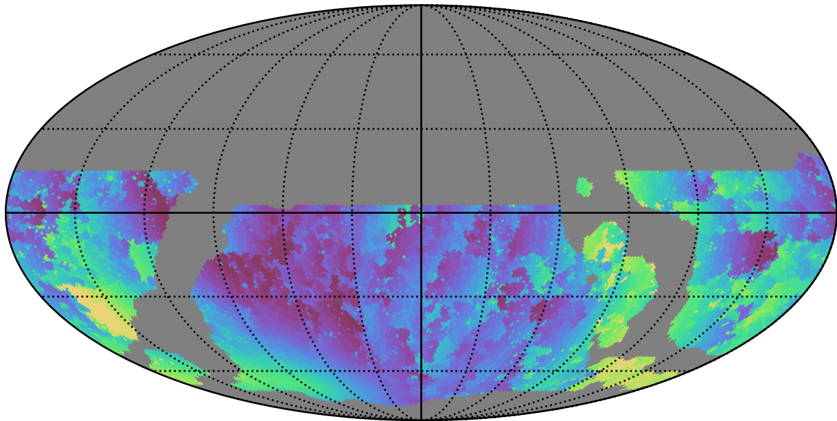
weather_cloudso36v3.4_10yrs WFD u band: Min solarElong
