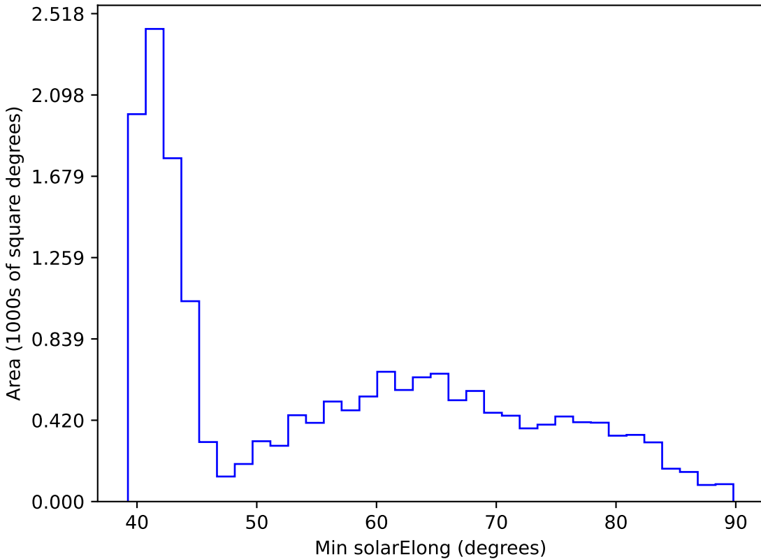
weather_cloudso36v3.4_10yrs WFD r band: Min solarElong
