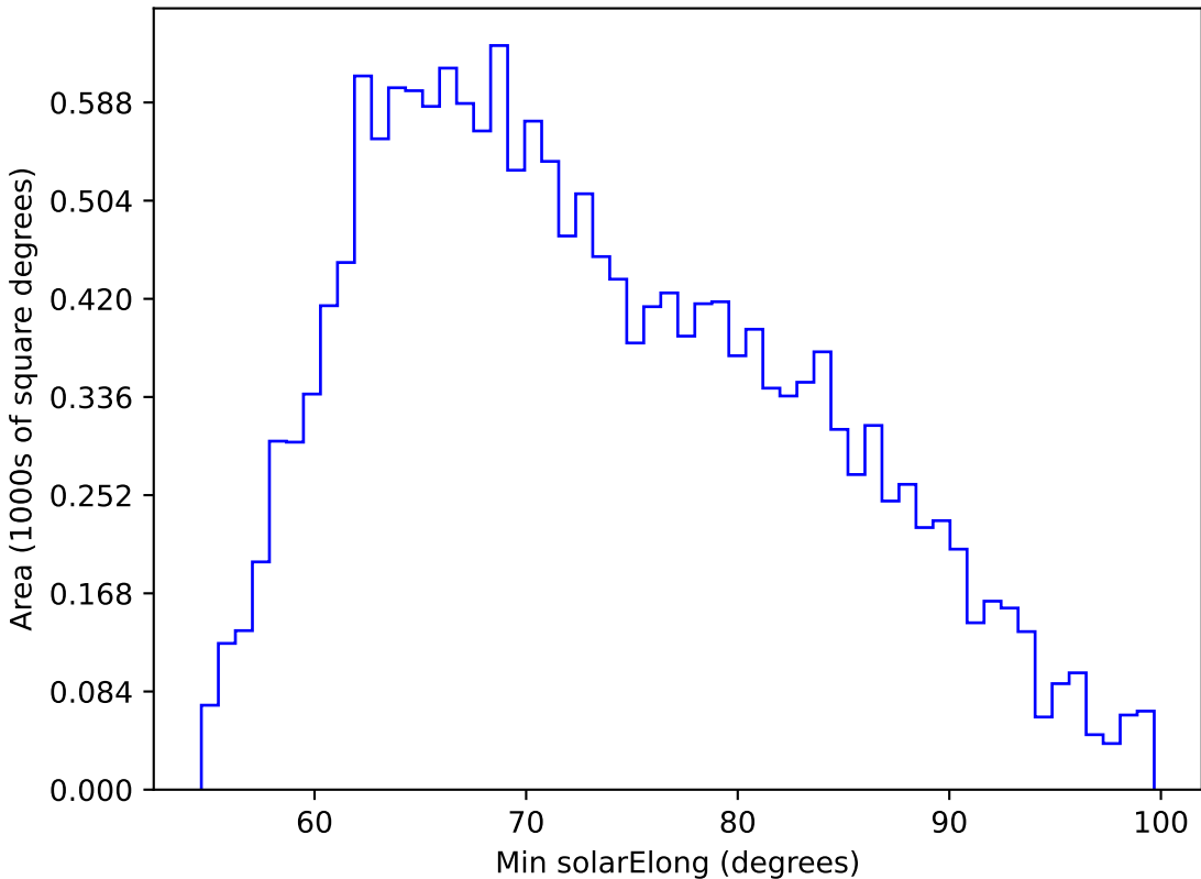
weather_cloudso36v3.4_10yrs WFD g band: Min solarElong
