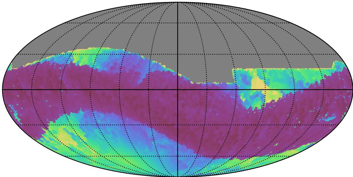
weather_cloudso36v3.4_10yrs All sky z band: Min solarElong
