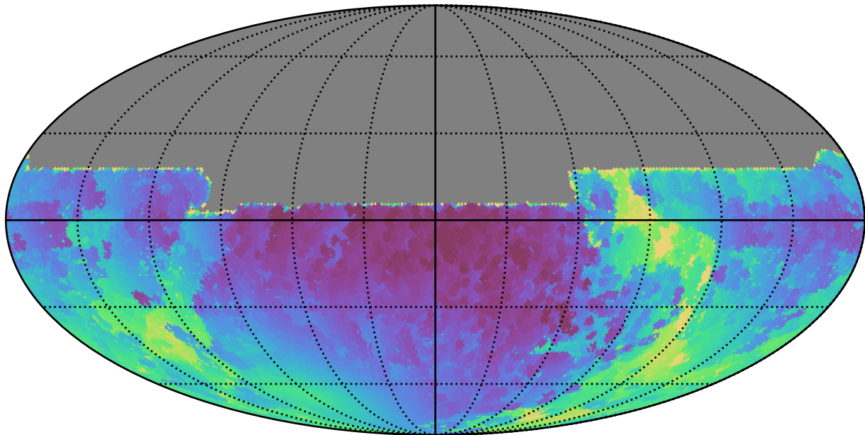
weather_cloudso36v3.4_10yrs All sky y band: Min solarElong
