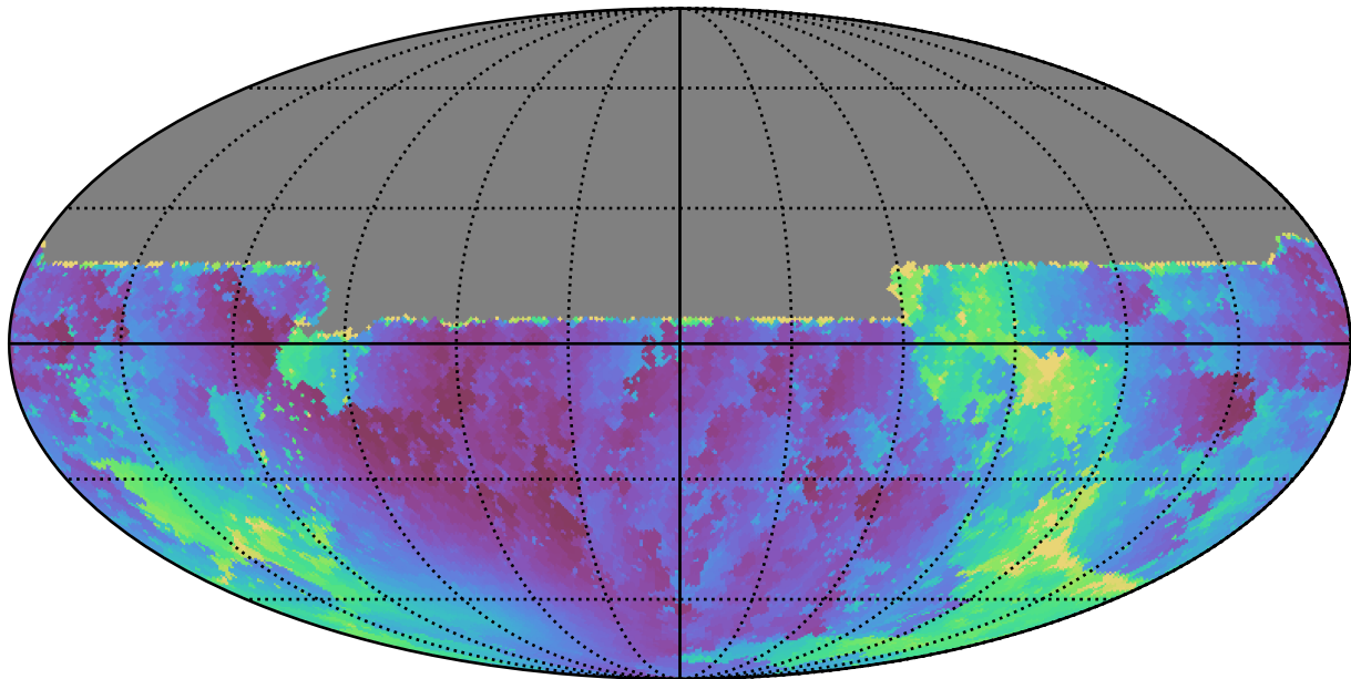
weather_cloudso36v3.4_10yrs All sky u band: Min solarElong
