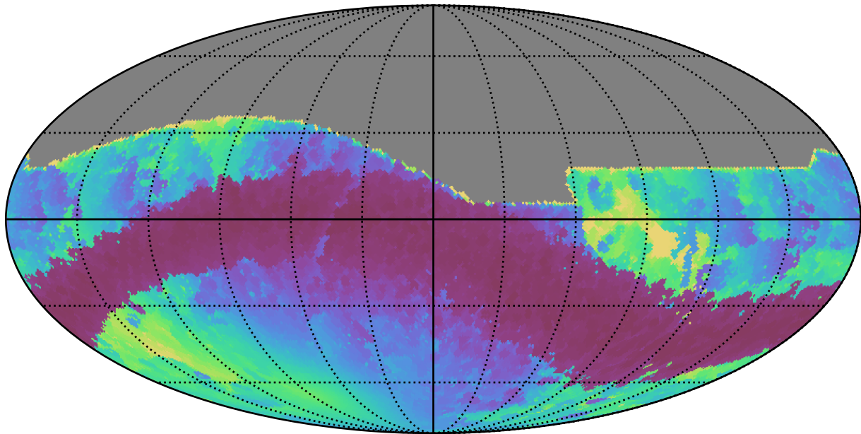
weather_cloudso36v3.4_10yrs All sky r band: Min solarElong
