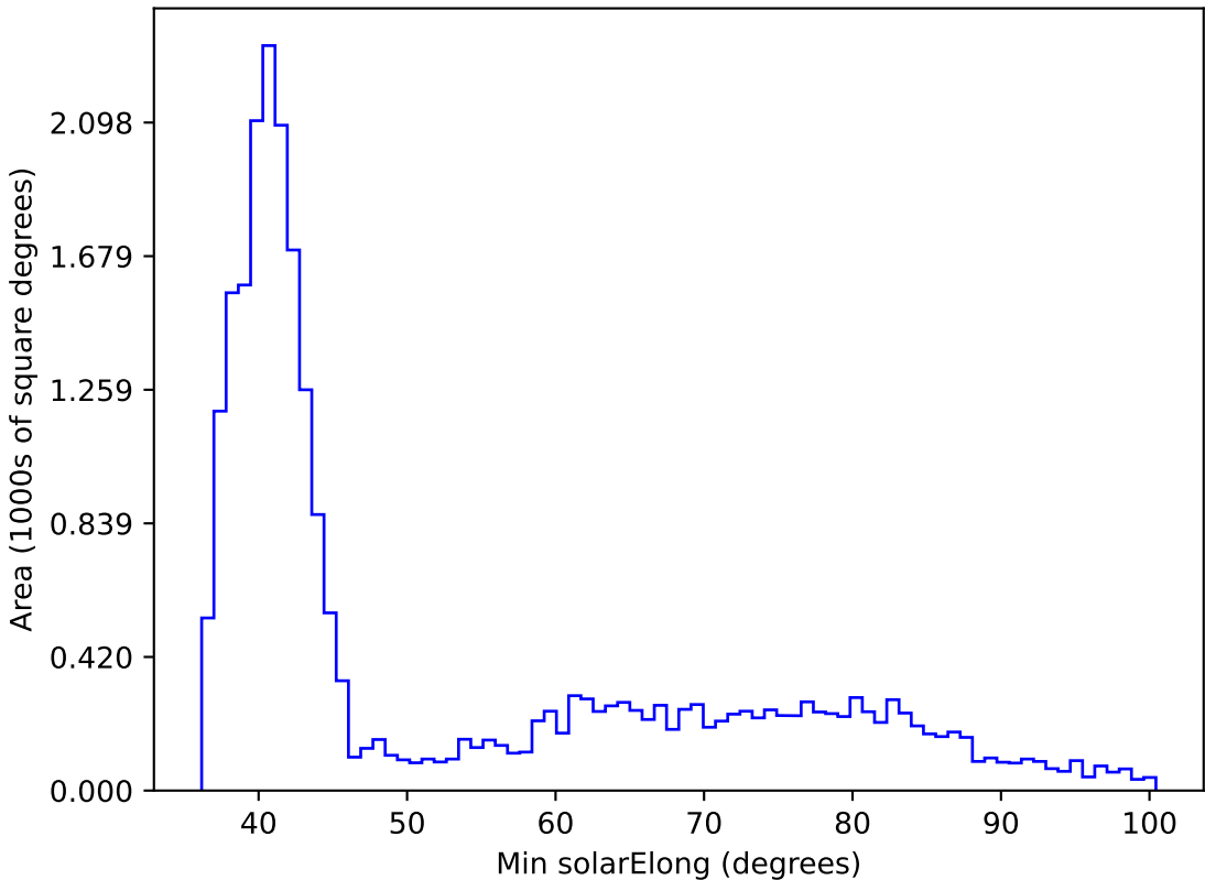
weather_cloudso36v3.4_10yrs All sky i band: Min solarElong
