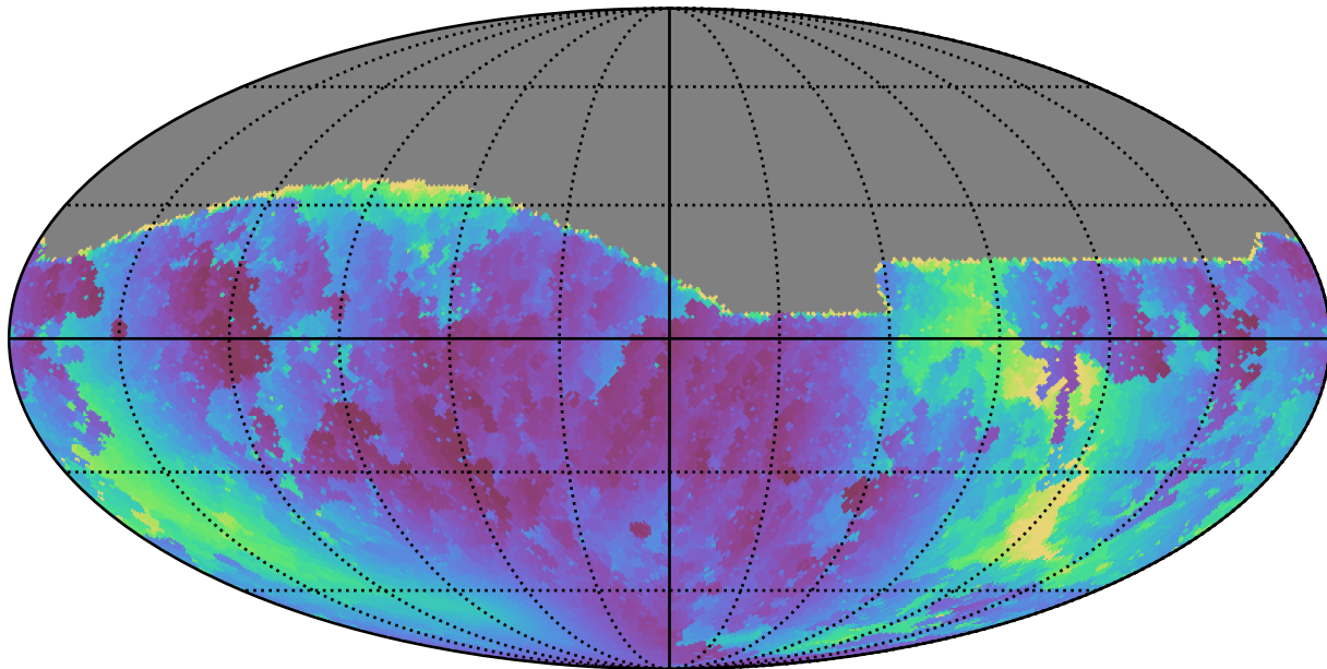
weather_cloudso36v3.4_10yrs All sky g band: Min solarElong
