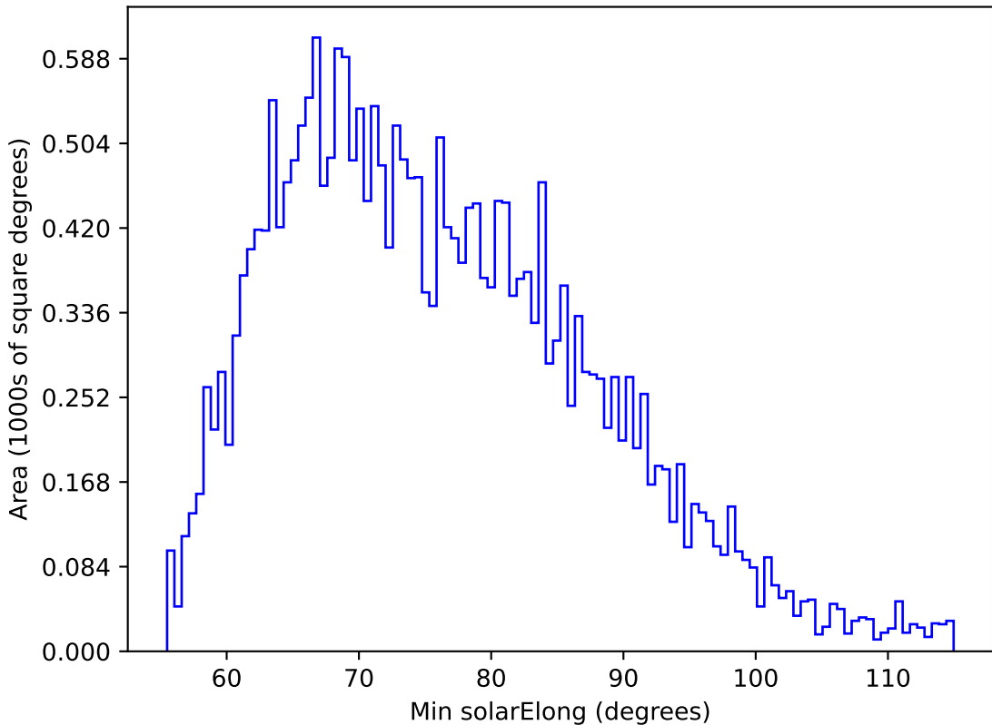
weather_cloudso36v3.4_10yrs All sky g band: Min solarElong
